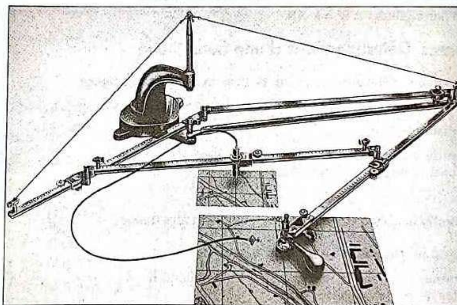
Un pantographe.
