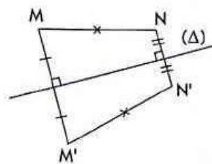
symétrie s_{\Delta} .
