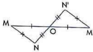
symétrie s_O .
